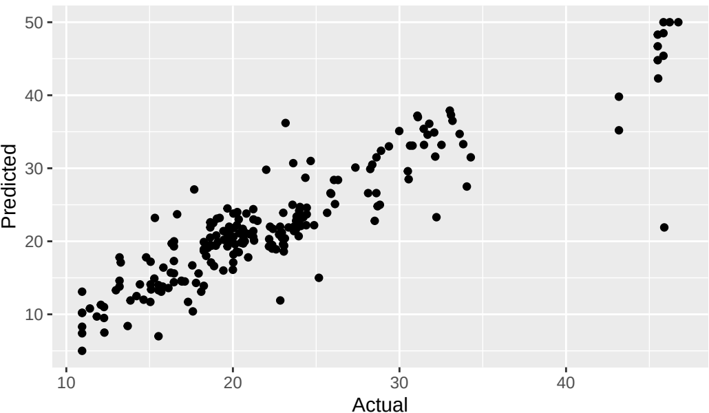
Bagging predicted vs actual
